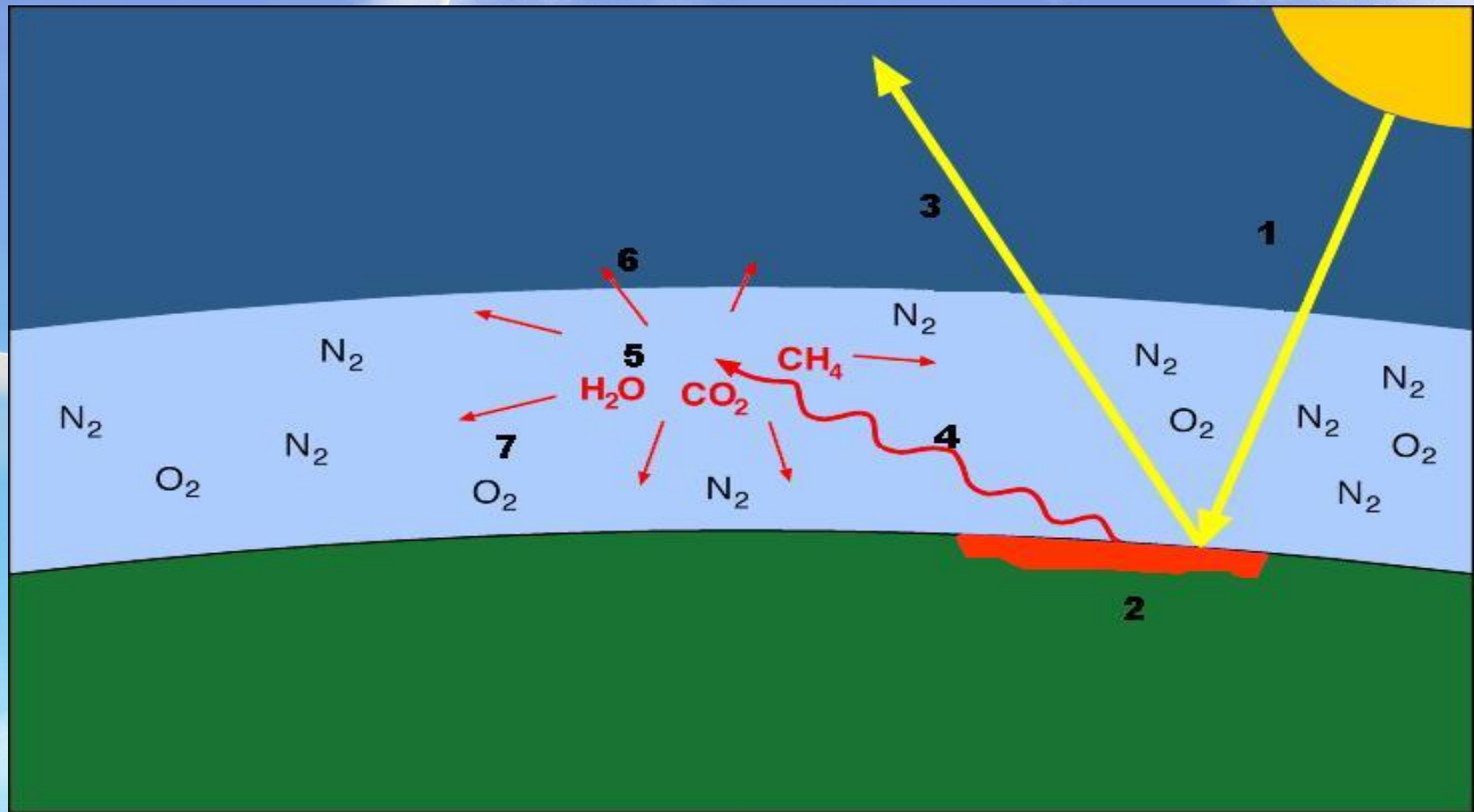
Schemat mechanizmu efektu cieplarnianego
